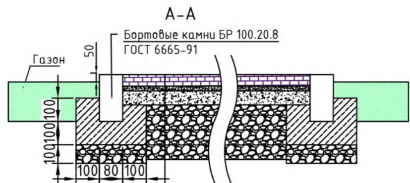
Устройство дорожной одежды тротуара (тип 1)
